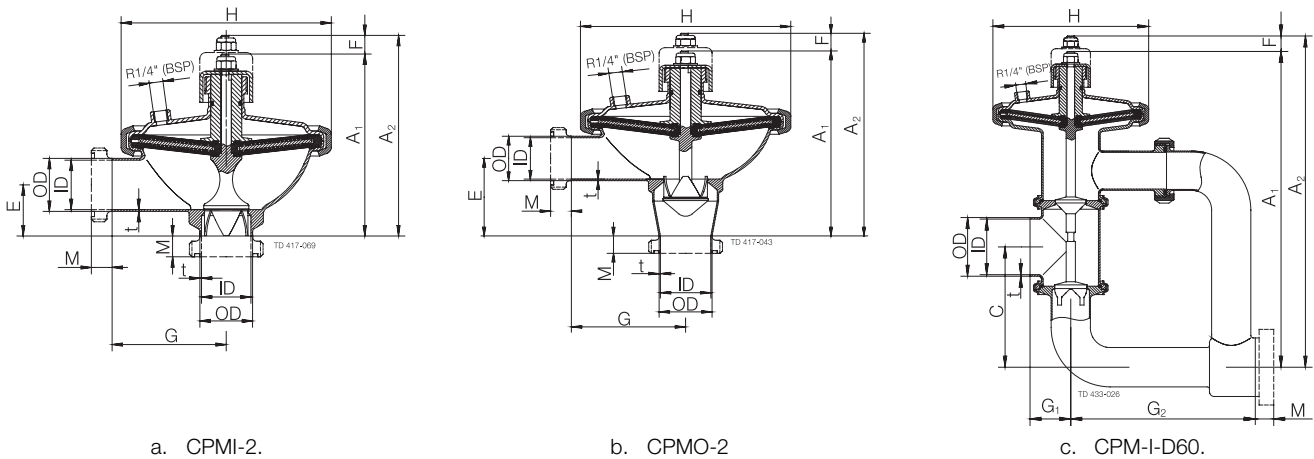
Fig. 2. Dimensions
